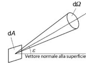
Schema della definizione di radianza.
