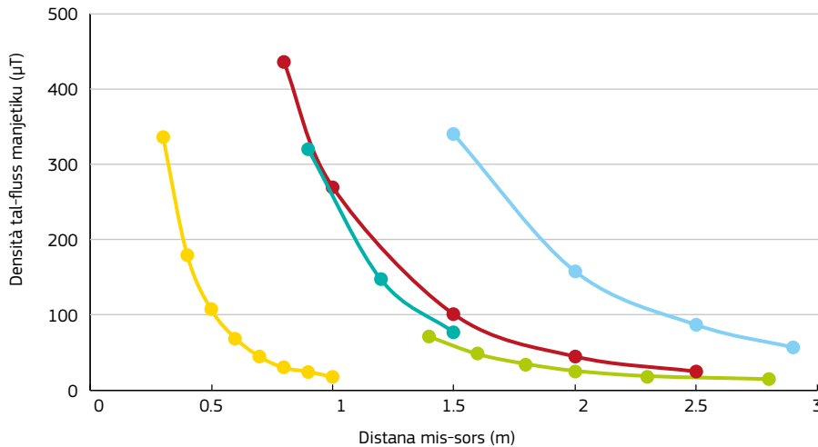
Figura 3.2. Tnaqqis fid-densità tal-fluss manjetiku skont id-distanza għal varjetà ta' sorsi ta' frekwenza tal-potenza: spot welder (●●); 0.5 m kojl demagnetizzatur (●●); 180 kW forn ta' induzzjoni (●●); 100 kVA seam welder (●●); 1 m demagnetizzazzjoni (●●)
