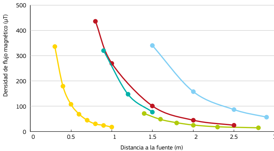
Figura 3.2. Disminución de la densidad de flujo magnético al aumentar la distancia a las fuentes de frecuencias con diferentes potencias: aparato de soldadura por puntos (●—●); bobina desmagnetizadora de 0,5 m (●—●); horno de inducción de 180 kW (●—●); aparato de soldadura en cordón de 100 kVA (●—●); bobina desmagnetizadora de 1 m (●—●)
