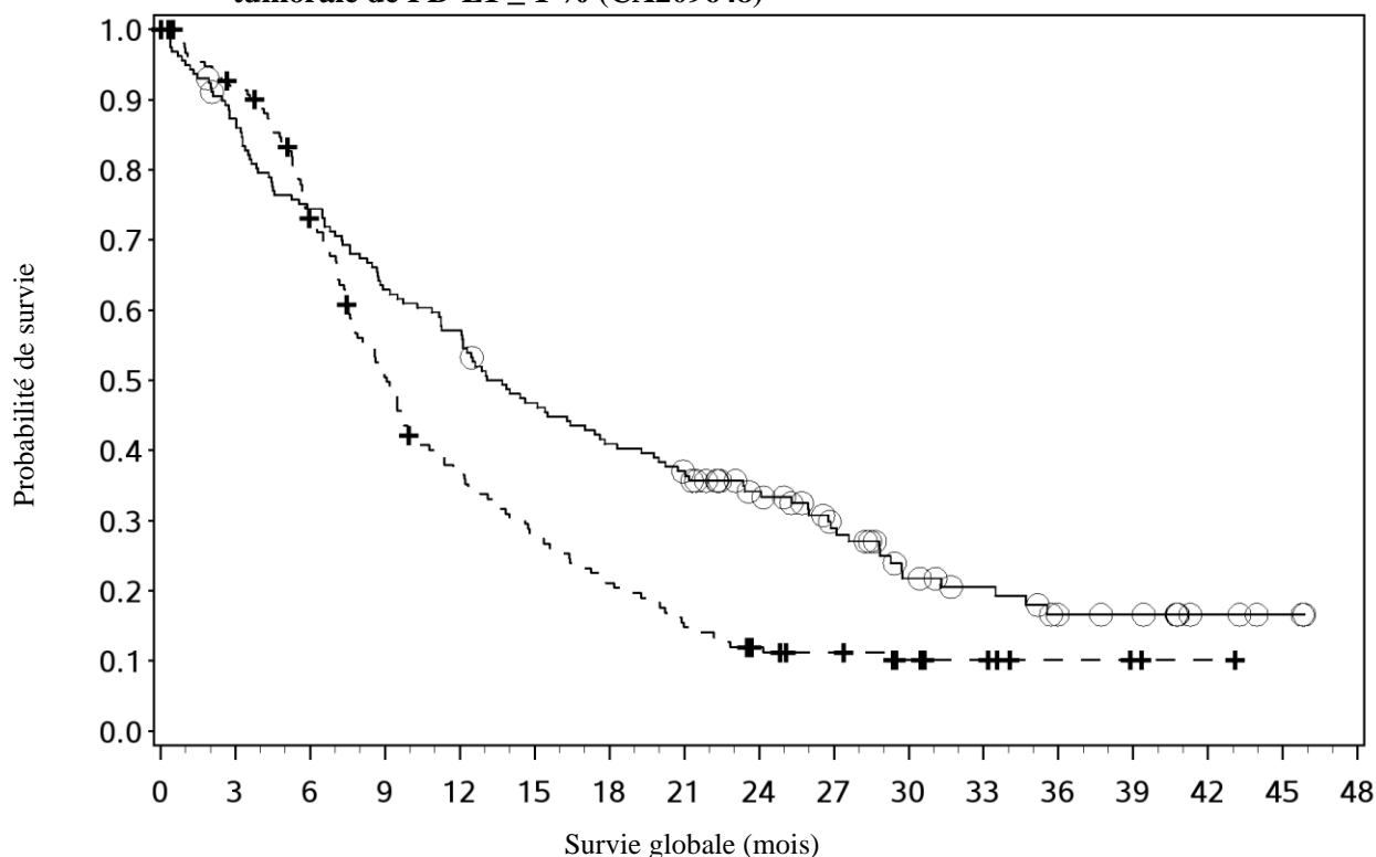
Figure 24 : Courbes de Kaplan-Meier pour la SG chez les patients présentant une expression tumorale de PD-L1 \geq 1 % (CA209648)
