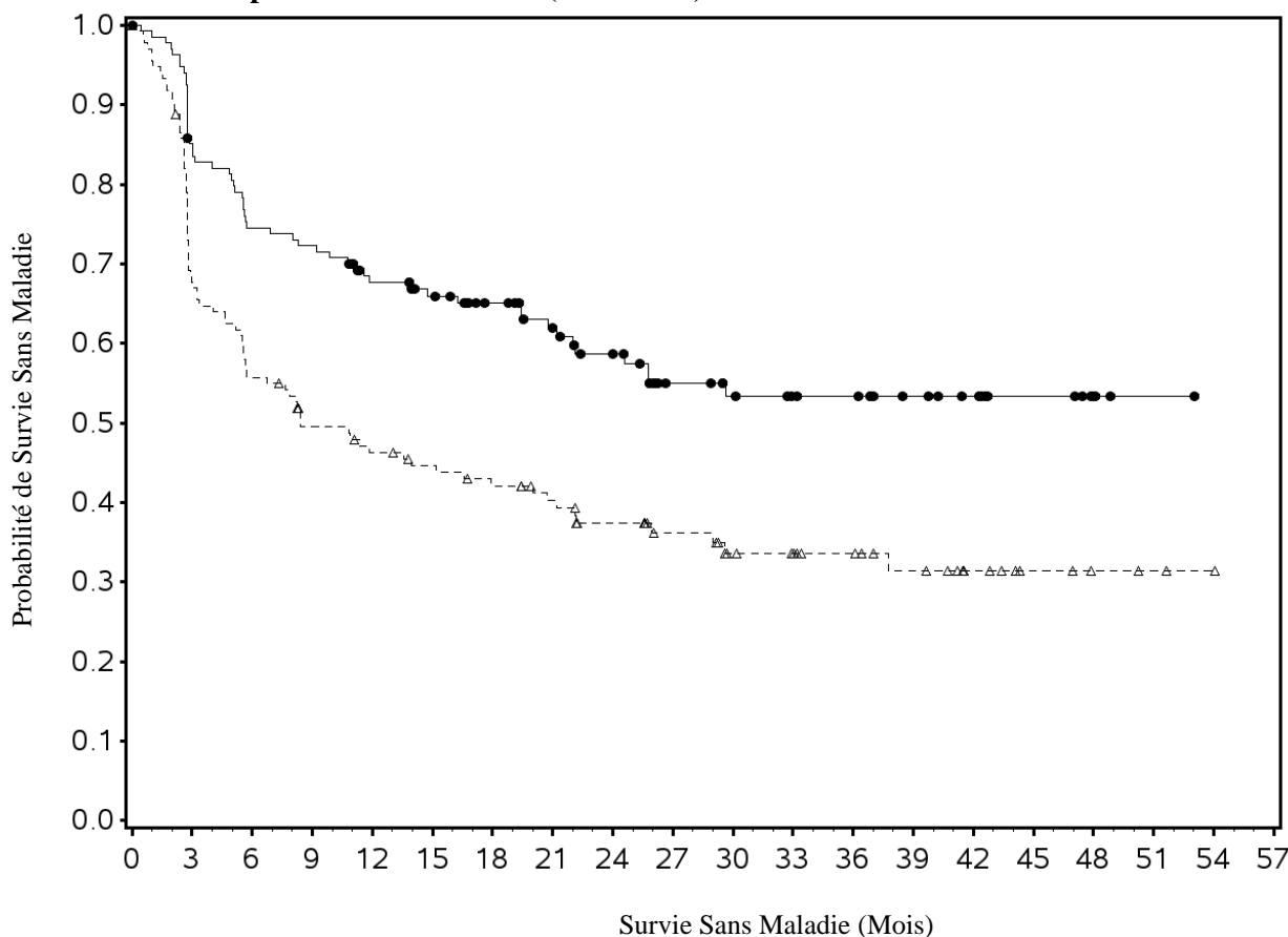
Figure 22 : Courbe de Kaplan-Meier de la SSM chez les patients avec des cellules tumorales exprimant PD-L1 \geq 1\% (CA209274)
