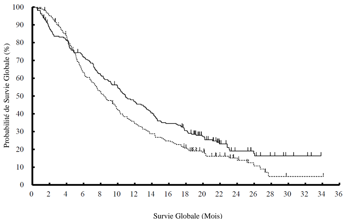
Figure 23 : Courbes de Kaplan-Meier de la SG (ONO-4538-24/CA209473)
