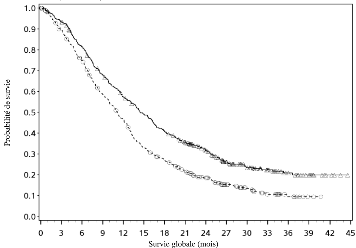
Figure 28 : Courbes de Kaplan-Meier pour la SG chez les patients PD-L1 avec un CPS \geq 5 (CA209649)
