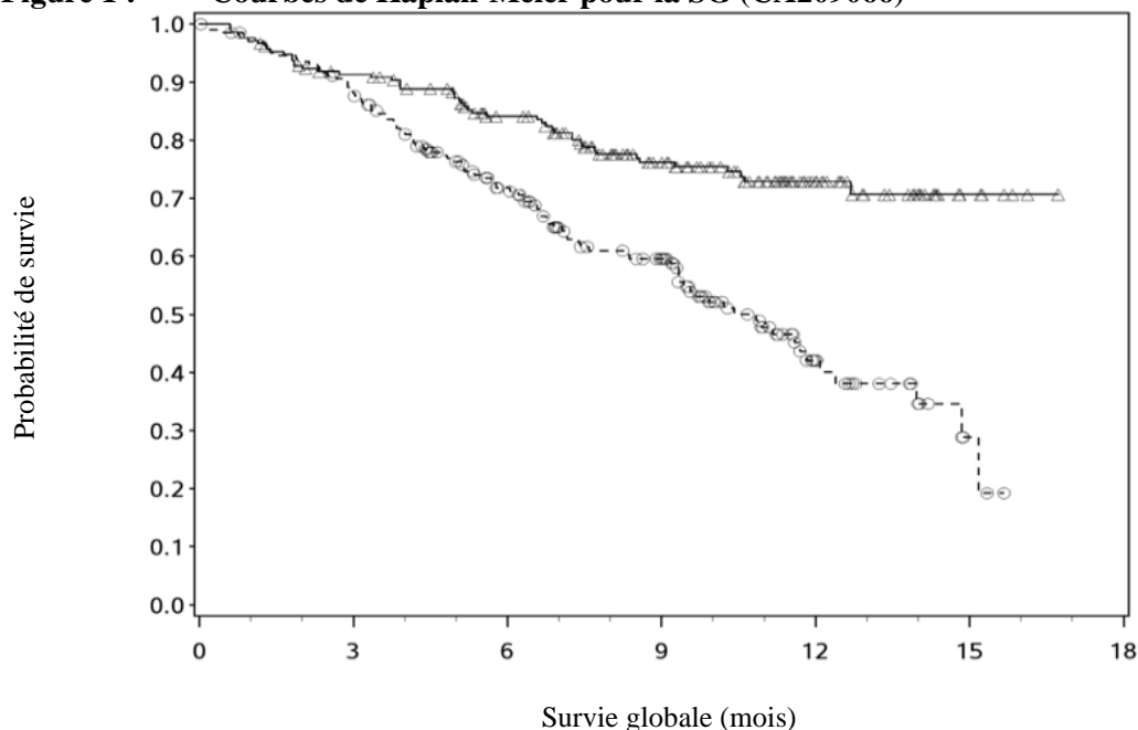
Figure 1 : Courbes de Kaplan-Meier pour la SG (CA209066)
