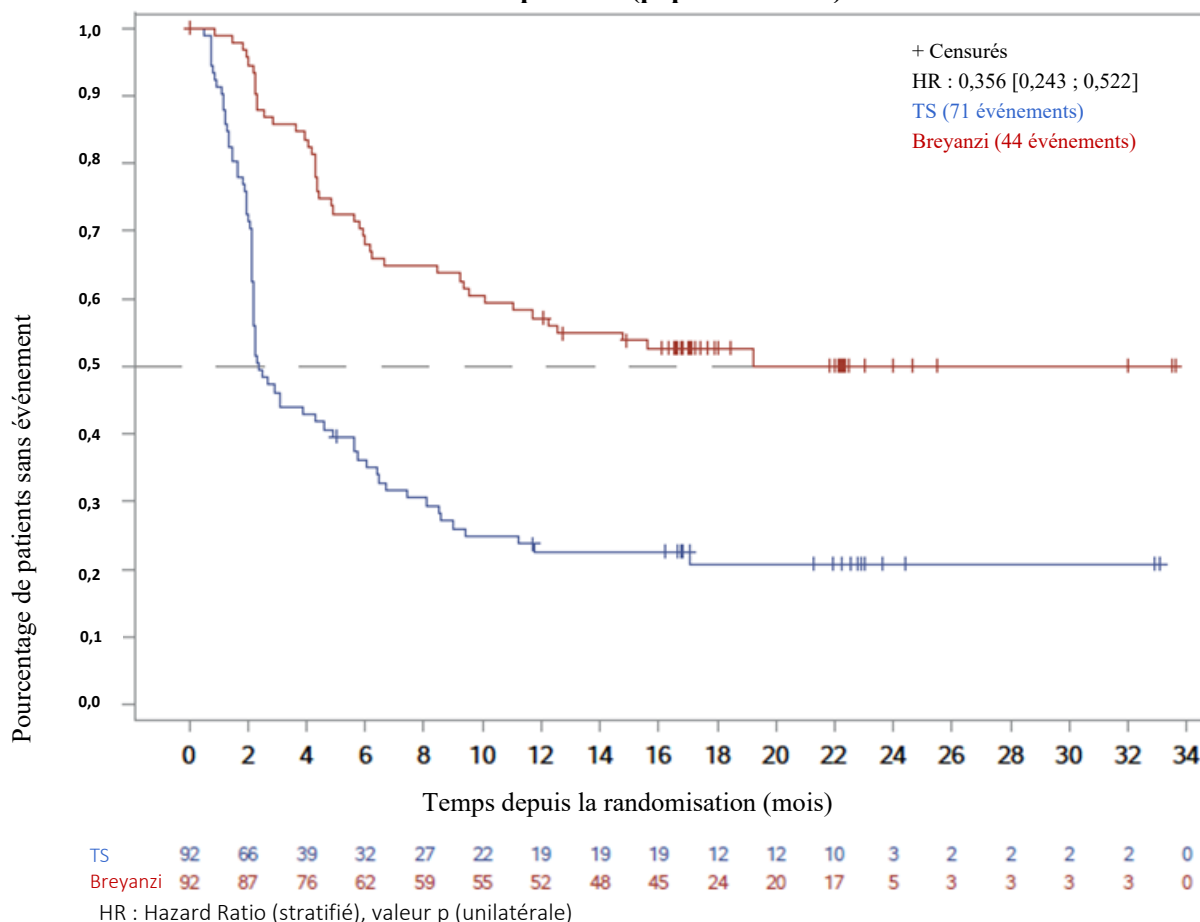
Figure 1. Courbe de Kaplan-Meier de la survie sans événement déterminée par le comité d'évaluation indépendant (population ITT)
