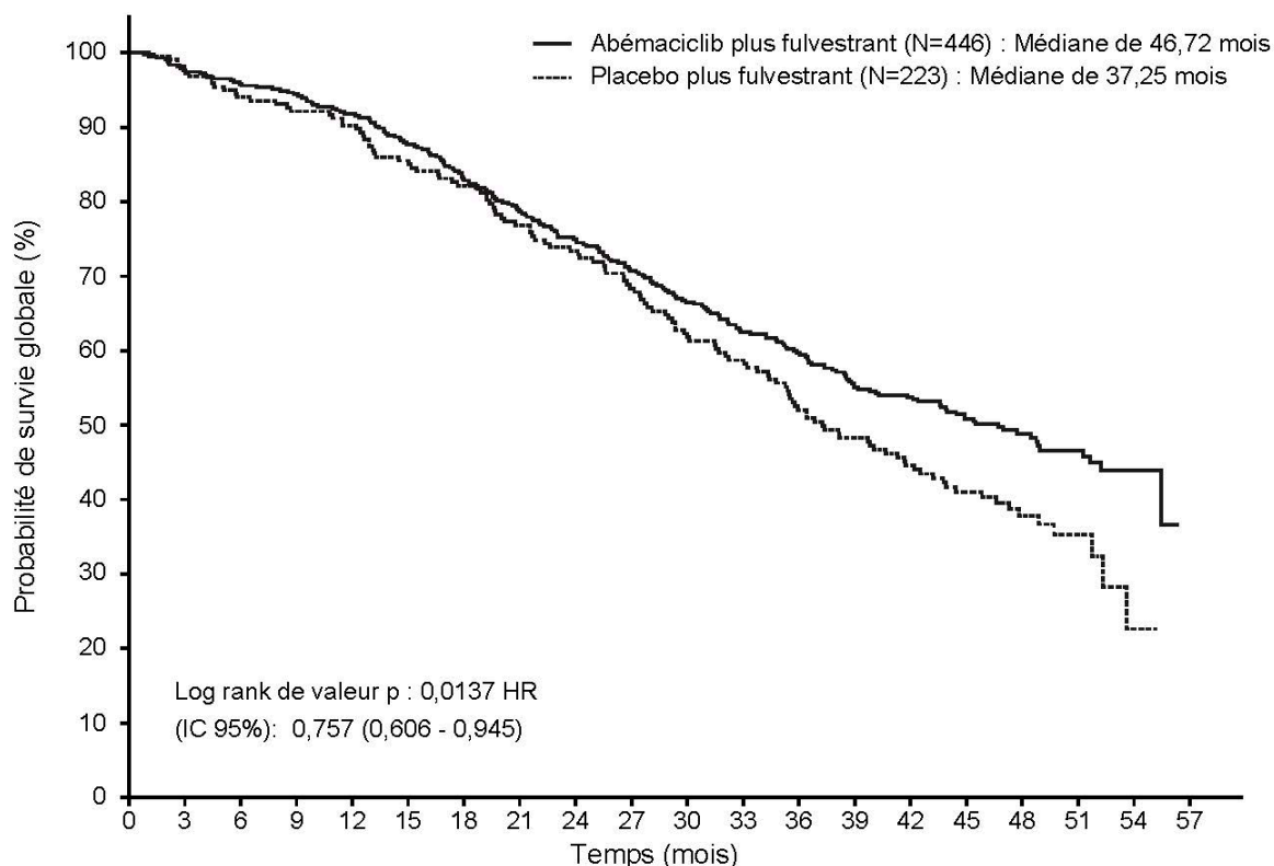
Figure 3. Etude MONARCH 2 : Courbe de Kaplan-Meier de la survie globale (Population en intention de traiter)
