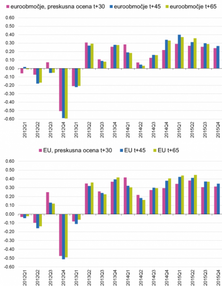
Slika 1: stopnje rasti (v %) za euroobmočje (zgornji grafikon) in EU (spodnji grafikon) pri t+30 (preskus), t+45 in t+65
