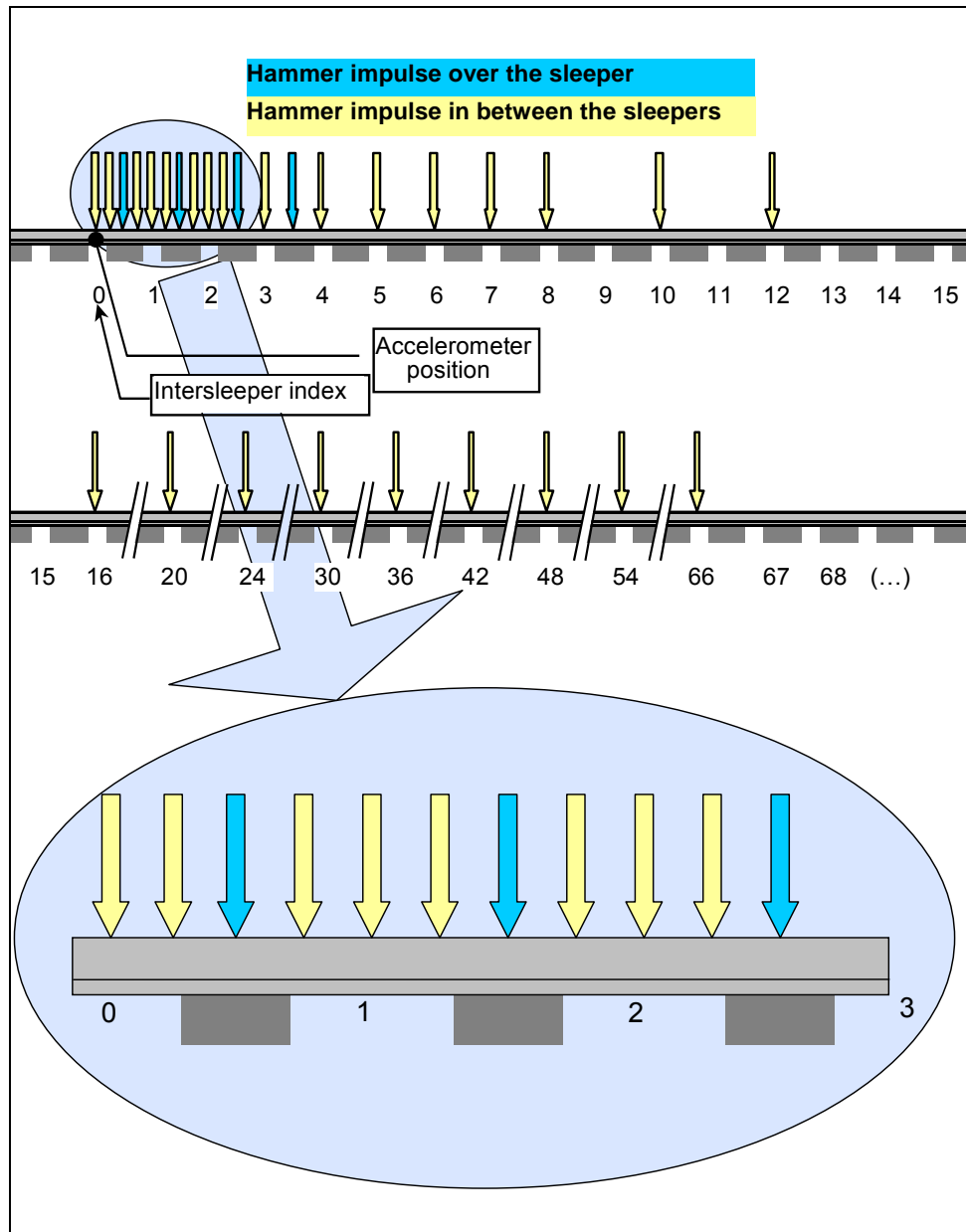
Bild F4: Dämpfungsraten - Anordnung der Erregungspunkte
