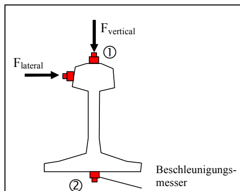
Bild F3: Anordnung der Beschleunigungsmesser an der Schiene (Querschnitt)
