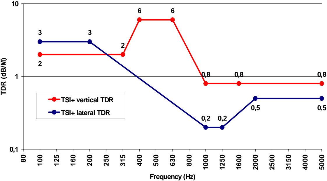
Bild F2: Vertikale und laterale Dämpfungsrate (TDR) - unteres Grenzwertspektrum des Referenzgleises
