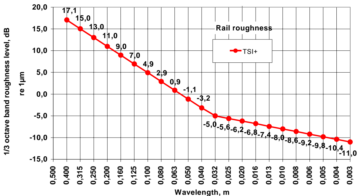
Bild F1: Schienenrauigkeit - Grenzwertspektrum des Referenzgleises
