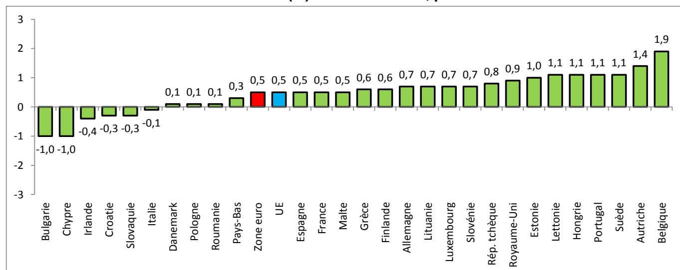
Taux d'inflation annuel (%) en octobre 2016, par ordre croissant
