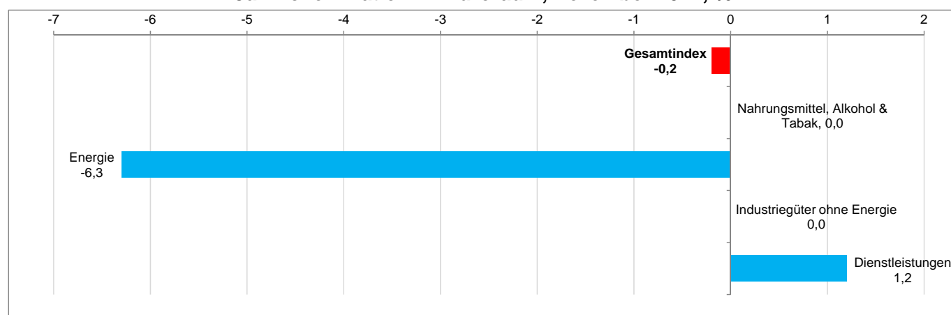
Jährliche Inflation im Euroraum, Dezember 2014, %
