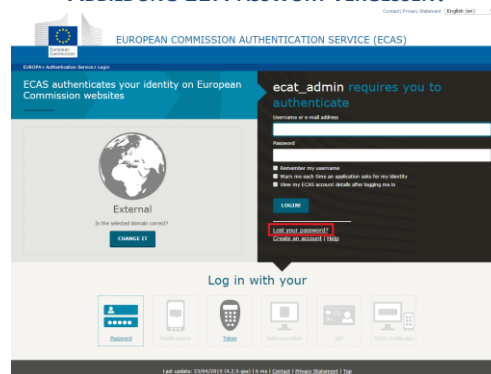
ABBILDUNG 11: PASSWORT VERGESSEN?
