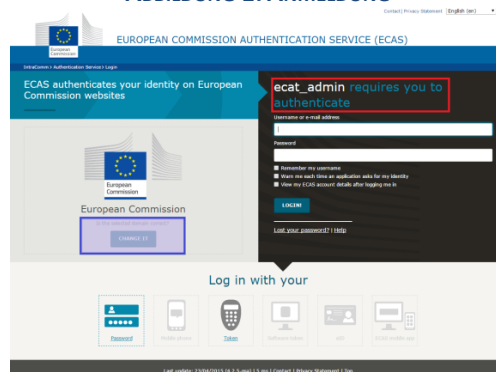
ABBILDUNG 1: ANMELDUNG
